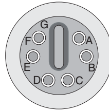
Figure 1-6 2150EX - Pinbelegung des Verbindungssteckers
